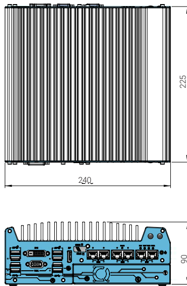
Nuvo-7000E/P
